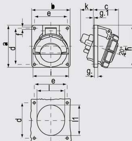
外形尺寸 Dimension
