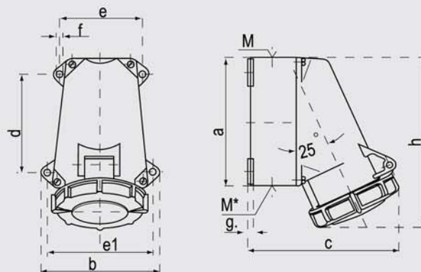
外形尺寸 Dimension
